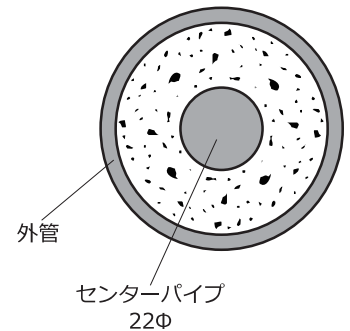
マッドチューブ 断面図
