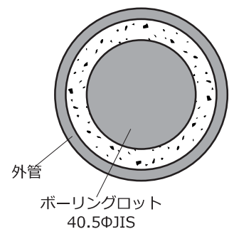
セジメントチューブ 断面図
